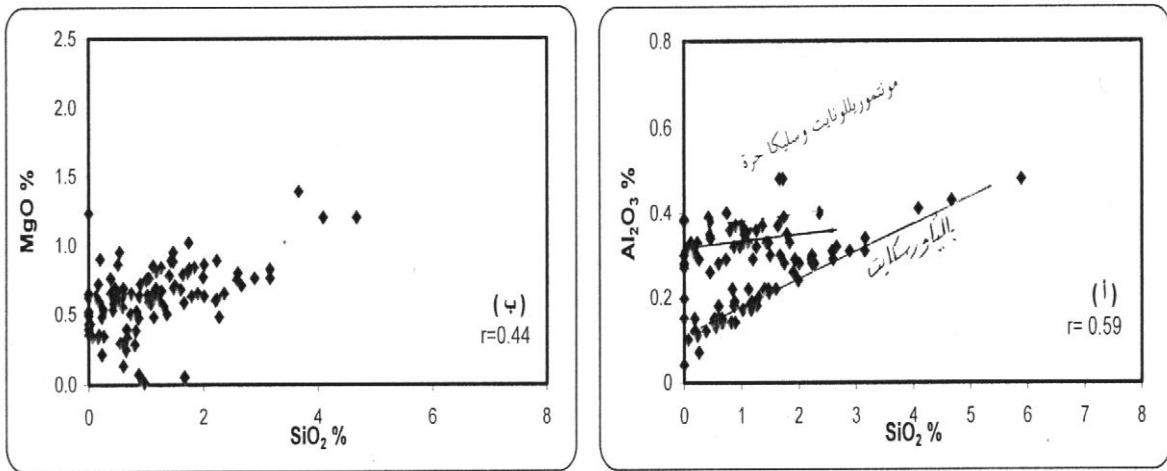
الشكل 3: علاقة السليكا مع الألومينا والمغنيسيا التي تعكس محتوى الفوسفورايت والصخور الجيرية الفوسفاتية المرافقة لها من المعادن الطينة الباليكورسكايت والمونتموريللوناييت.
